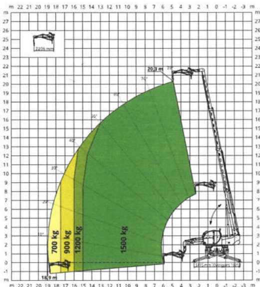
JIB MIT SEILWINDE 1.500 kg
