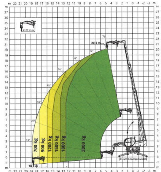
JIB MIT SEILWINDE 2.000 kg
