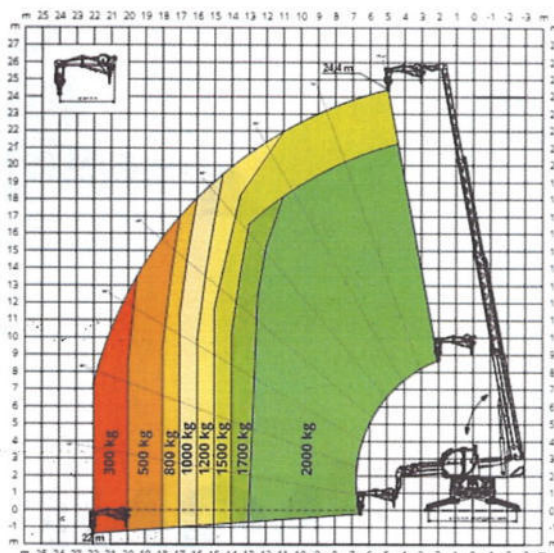
JIB MIT SEILWINDE 2.000 kg
