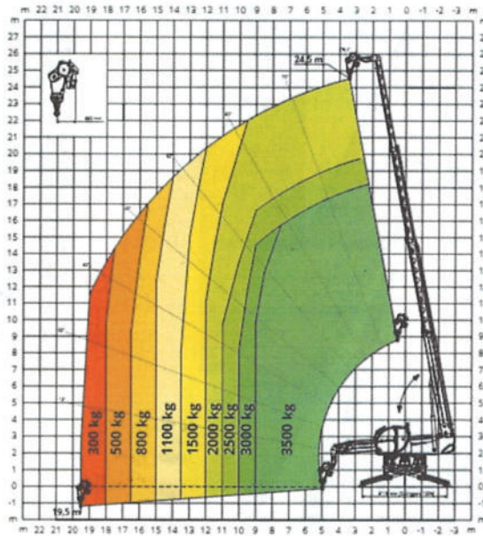
JIB MIT SEILWINDE 1.500 kg
